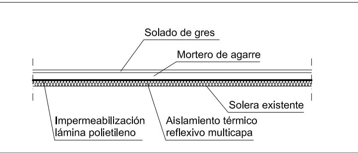
Detalle 2 _____
