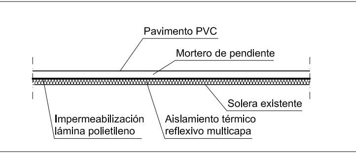
Detalle 3 _____
