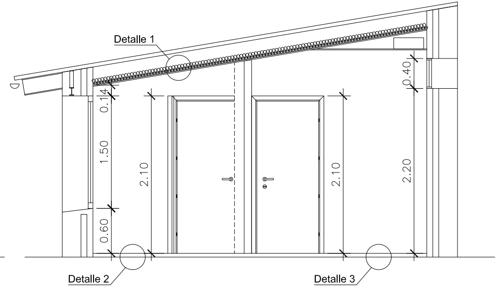
SECCIÓN 1-1' _____
